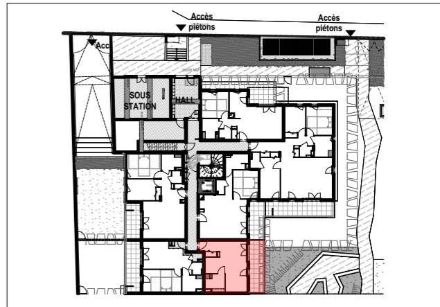
PLAN ETAGE
